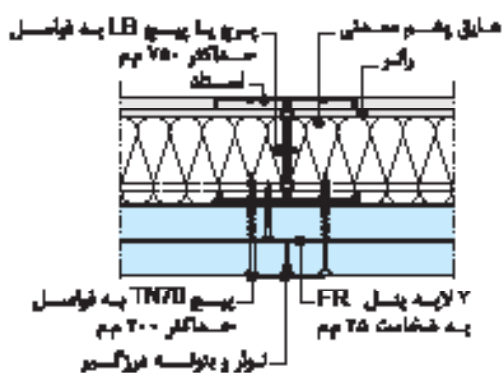
فرز قسام (F90)
