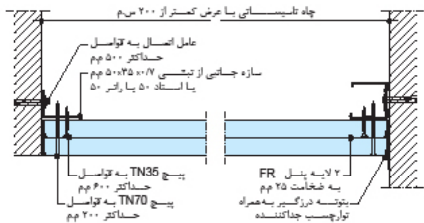
اتصال به دیوار بنایی جانبی
