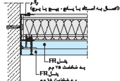
اتصال به دیوار پلاستیکی چغنی (F60)
