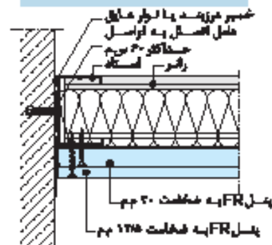
اتصال به دیوار بتنی چسبی (F30)
