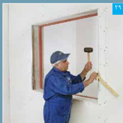
۲۹ تنظیم پتل نواری (گونیا کردن)
