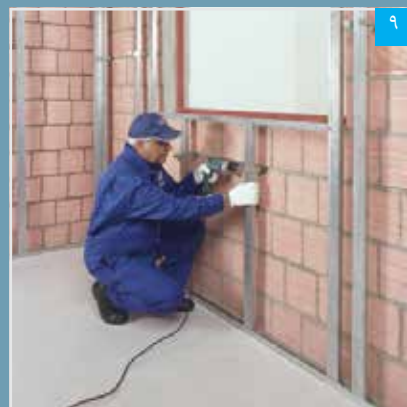
۹ اتصال سازه های قائم به براکت‌ها
