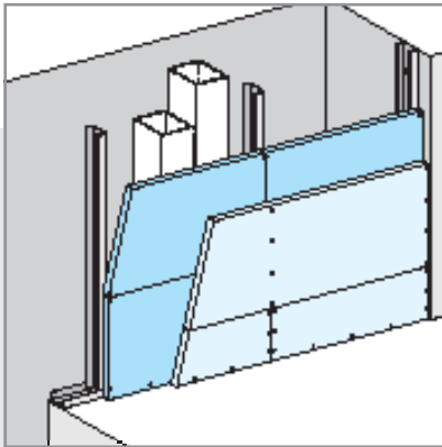
دیوار پوششی W628b (پوشش کاری ۲۵×۲ م.م)
