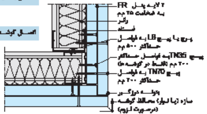
اتصال به دیوار بتنی یا سانی چسبی
