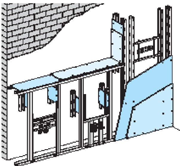
دیوار پوششی تأسیساتی (اجرا به صورت موضعی و با ارتفاع محدود)
