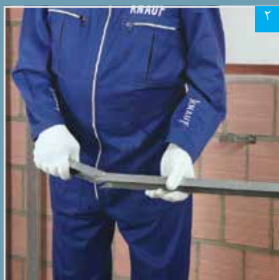
۲ خم کردن سازه برش خورده
