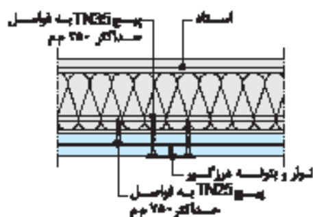
هرز قائم (F30)
