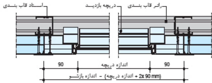
جزئیات نصب دریچه بازدید
