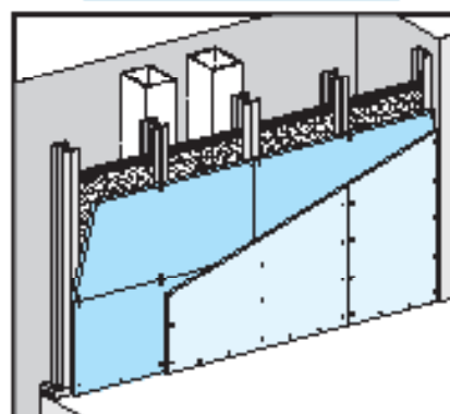
دیوار پوششی W629 (F60: پوشش کاری ۲۰x۱۲/۵ م.م) لایه اول افقی و لایه دوم عمودی تعبیه می‌شود
