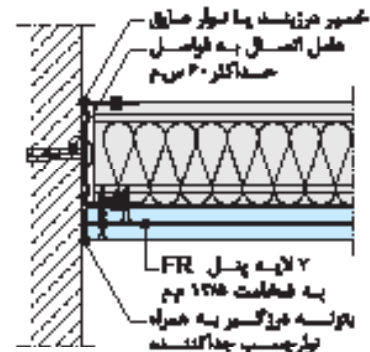
اتصال به دیوار پلاستیکی چغنی (F30)
