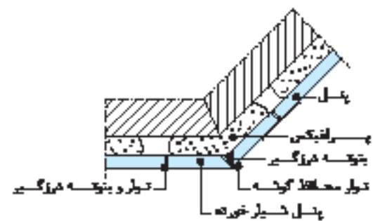
اتصال گوشه ۱۳۵ درجه
