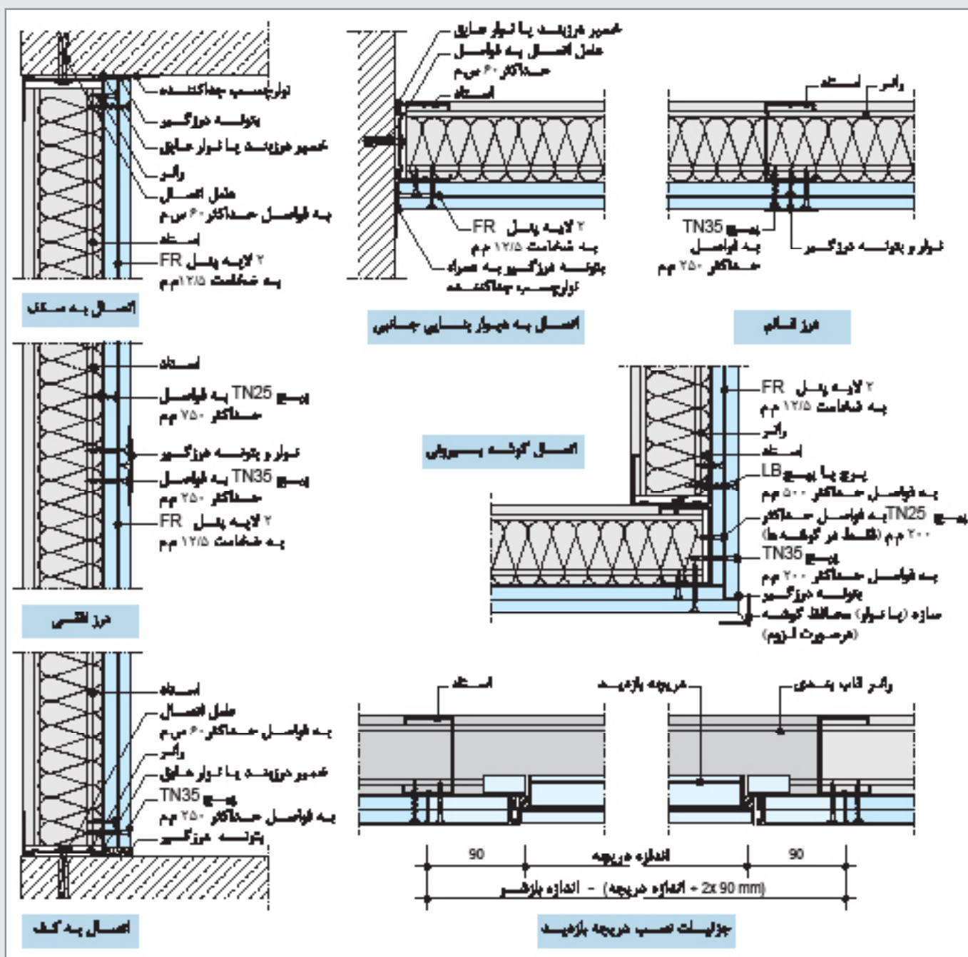
دیوار پوششی W628b (پوشش کاری ۲×۱۲/۵ م.م)
