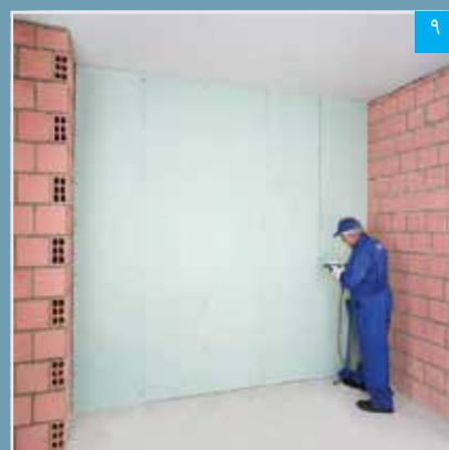
۹ نصب لایه دوم پنل ها و تکمیل ساختار
