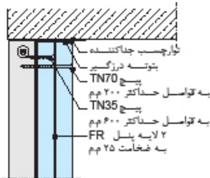
اتصال به سقف
