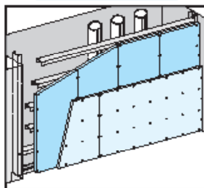
دیوار پوششی W630 (F60): پوشش کلری ۲۵x۱۸ (م.م) لایه اول عمودی و لایه دوم افقی تعبیه می‌شود
