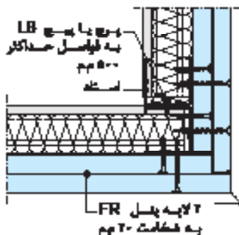
اتصال گوشه پیروزی (F90)
