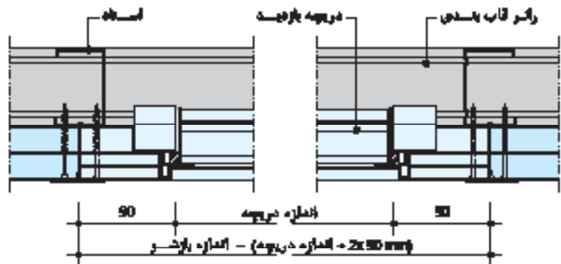
چگونگی نصب دریچه بارش
