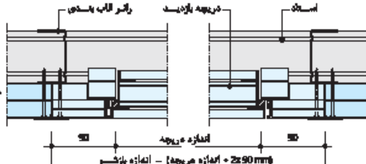
جزئیات نصب دریچه بازدهنده
