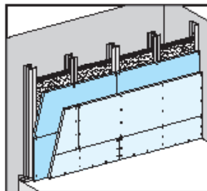
دیوار پوششی W629 (F90: پوشش کاری ۲۰x۲۵ م.م) هر دو لایه افقی تعبیه می‌شود
