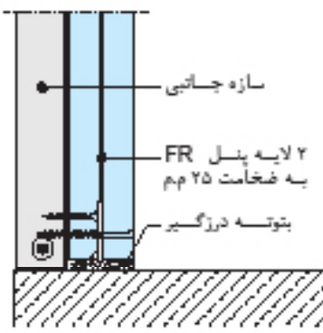
اتصال به کف
