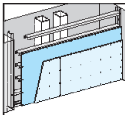
دیوار پوششی W630 (F30): پوشش کلری ۲۵x۱۲۵ (م.م) هر دو لایه افقی تعبیه می‌شود
