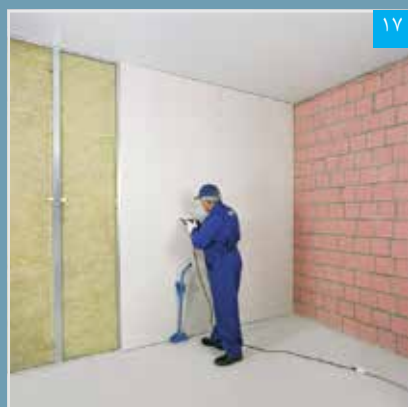
۱۷ نصب پنل‌ها
