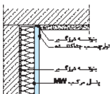
اتصال تازک کاری سقف به پوشش کاری
