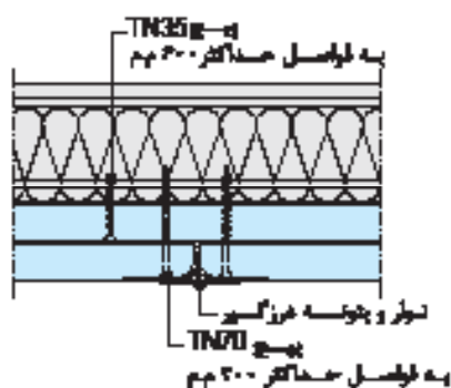
هرز قائم (F90)
