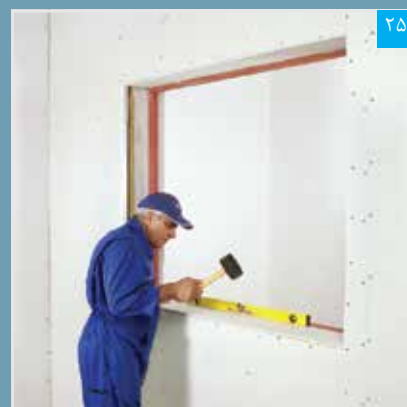
تنظیم پنل نواری (تراز کردن)
