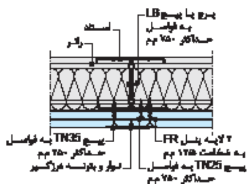
فرز قسام (F30)
