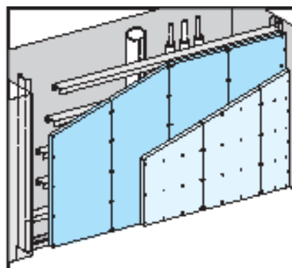
دیوار پوششی W630 (F90): پوشش کلری ۲۵x۲۵ (م.م) هر دو لایه عمودی تعبیه می‌شود
