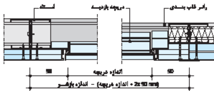
جزئیات نصب درجه پوزید (F30)
