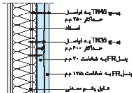
اتصال به دیوار بتنی چسبی (F60)
