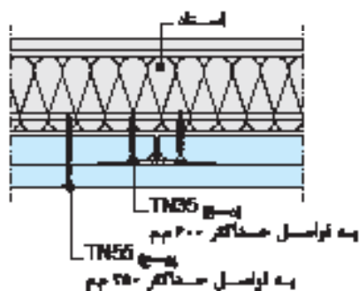
هرز قائم (F60)
