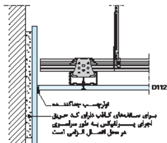
اتصال سقف کلاف به پوشش کاری
