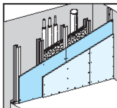
دیوار پوششی W629 (F30: پوشش کاری ۲۰x۱۲/۵ م.م) هر دو لایه عمودی تعبیه می‌شود
