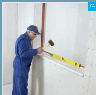
۳۵ نصب و تنظیم سنگ کف پنجره
