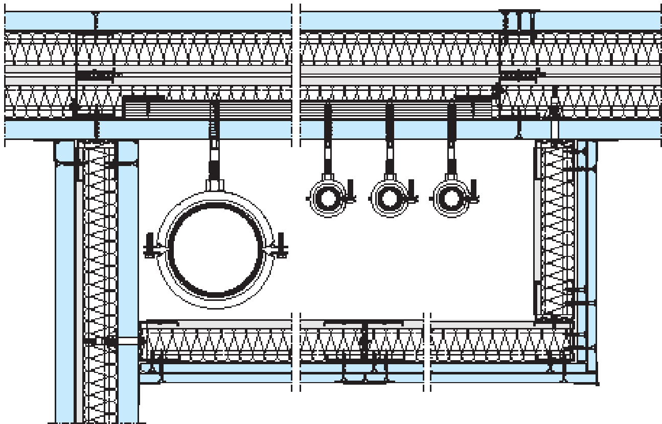
دیوار چاه تأسیساتی
