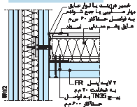
اتصال به دیوار بتنی چسبی (F90)
