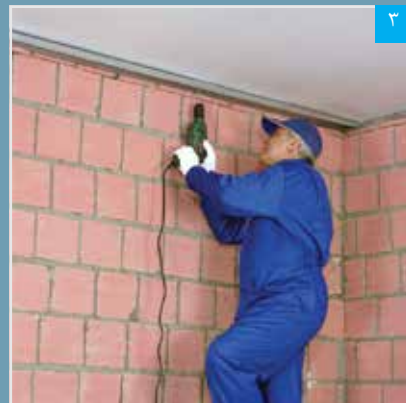
نصب رانر سقف
