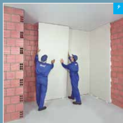
۶ استقرار پنل بر روی دیوار زمینه
