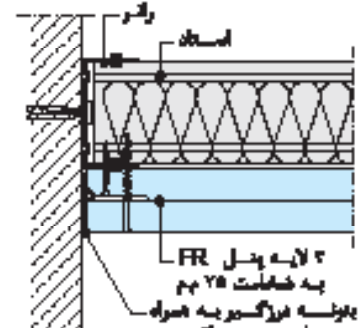
اتصال به دیوار پلاستیکی چغنی (F90)
