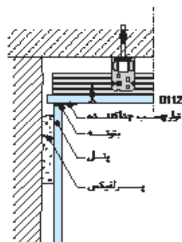
اتصال پوشش کاری به سقف کلاف
