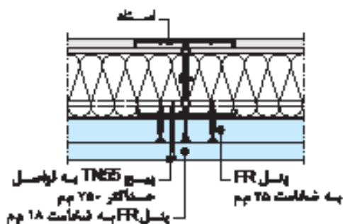
فرز قسام (F60)
