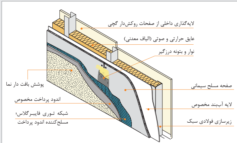
دیوار جداکننده خارجی
