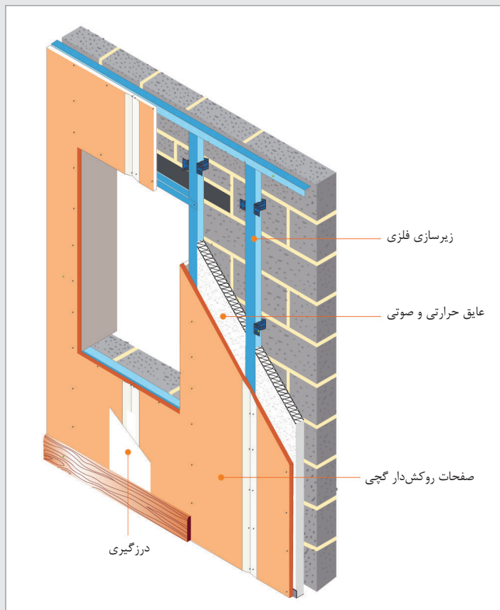
دیوار پوششی با سازه
