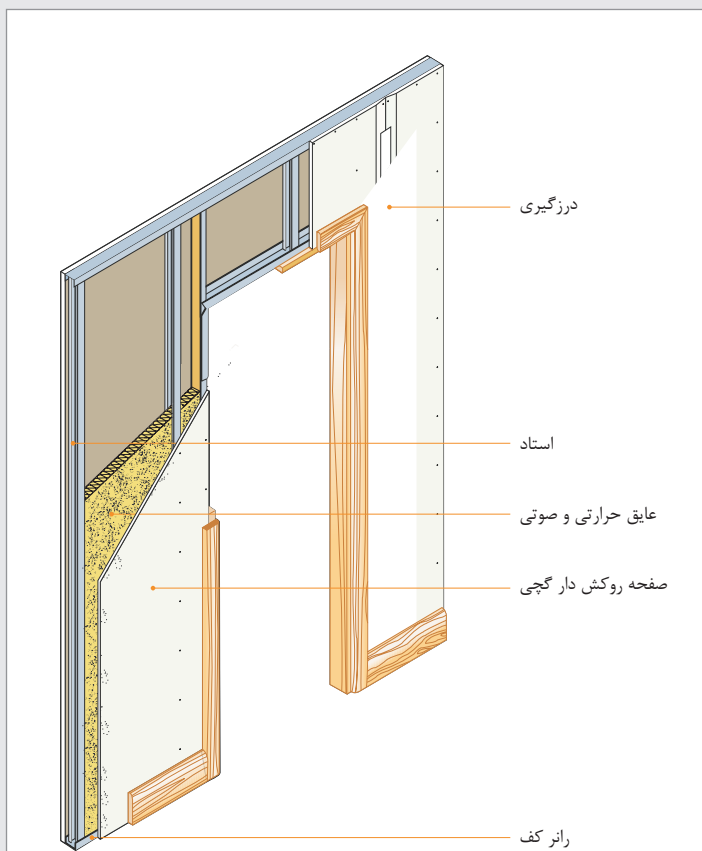
دیوار جداکننده داخلی
