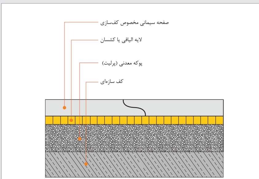
کف شناور
