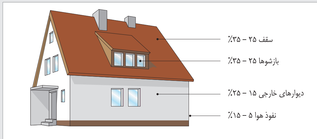
درصد نفوذ گرما در پوسته ساختمان‌ها - تابستان
