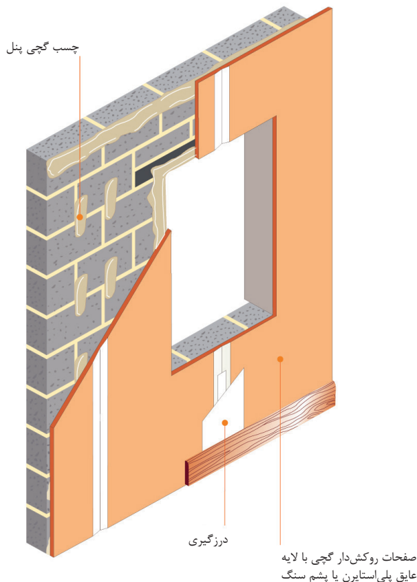
دیوار پوششی بدون سازه
