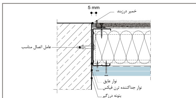
W384E-A1 اتصال به دیوار با مصالح بنایی
