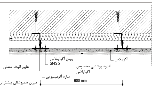
W684T-SO - V2 سطح مقطع افقی
