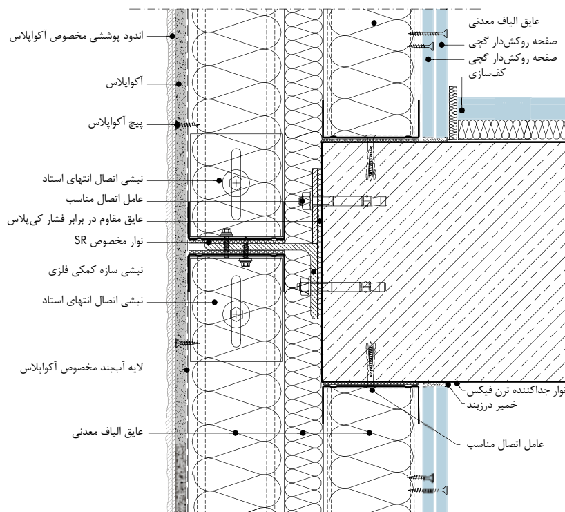
W388E-VM2 گزینه ۲: اتصال به سقف در تراز طبقات با استفاده از ورق و نبشی فولادی
