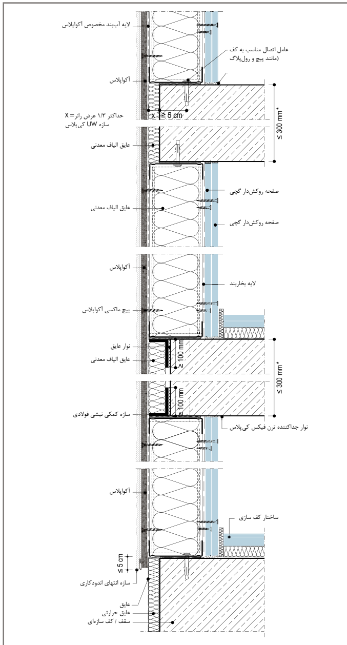
W384E-V2 گزینه ۲: مقطع عمودی
