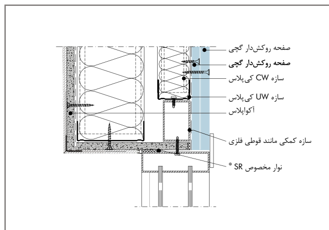
W388E-FE - VO2 گزینه ۲: اتصال دیوار خارجی آکوپالاس به قاب بالای پنجره
