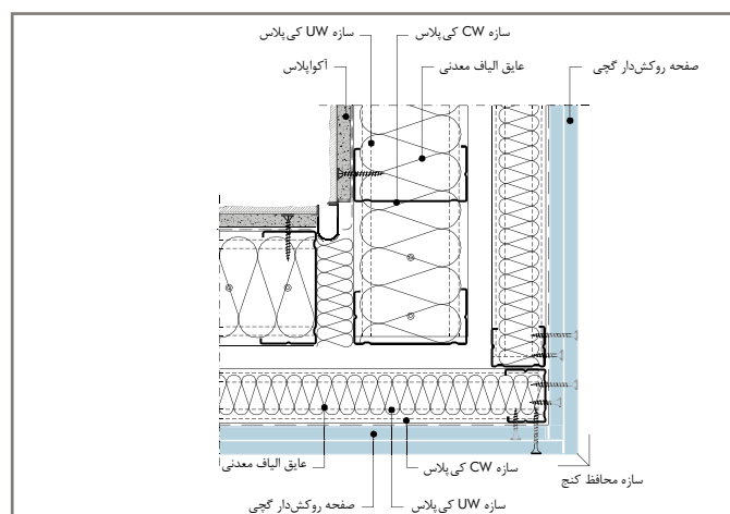
W388E-DBFU1 اتصال کنج داخلی به همراه سازه درز انقطاع
