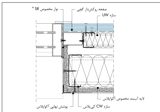
W388E-FE - VM1 گزینه ۱: پلان اتصال دیوار خارجی به پنجره
