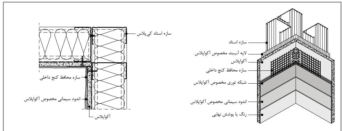
اتصال کنج داخلی با سازه PVC مخصوص
