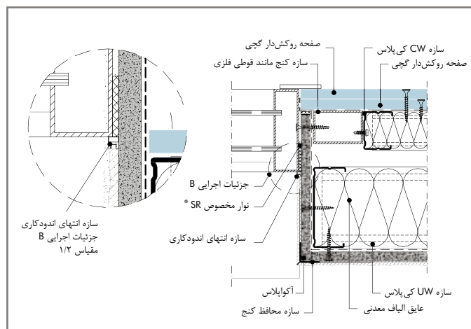
W388E-FE - VM2 گزینه ۲: پلان اتصال دیوار خارجی به پنجره
