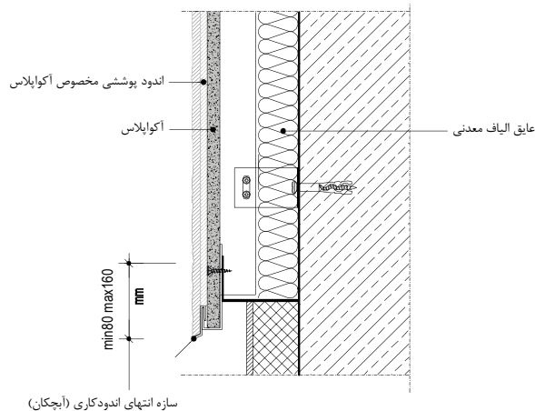
W684T-SO - V1 گزینه ۱: قسمت انتهایی کار در نما (نقطه شروع)
