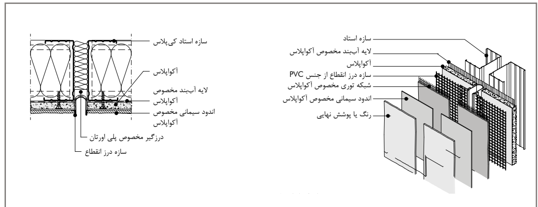
درز انقطاع با سازه PVC مخصوص
