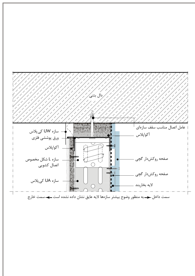
W384E-VOG1 گزینه ۱: اتصال کشویی لغزان به سقف سازه‌ای
