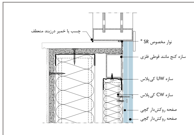
W388E-FE - VU2 گزینه ۲: اتصال دیوار خارجی آکوپالاس به قاب پایین پنجره
