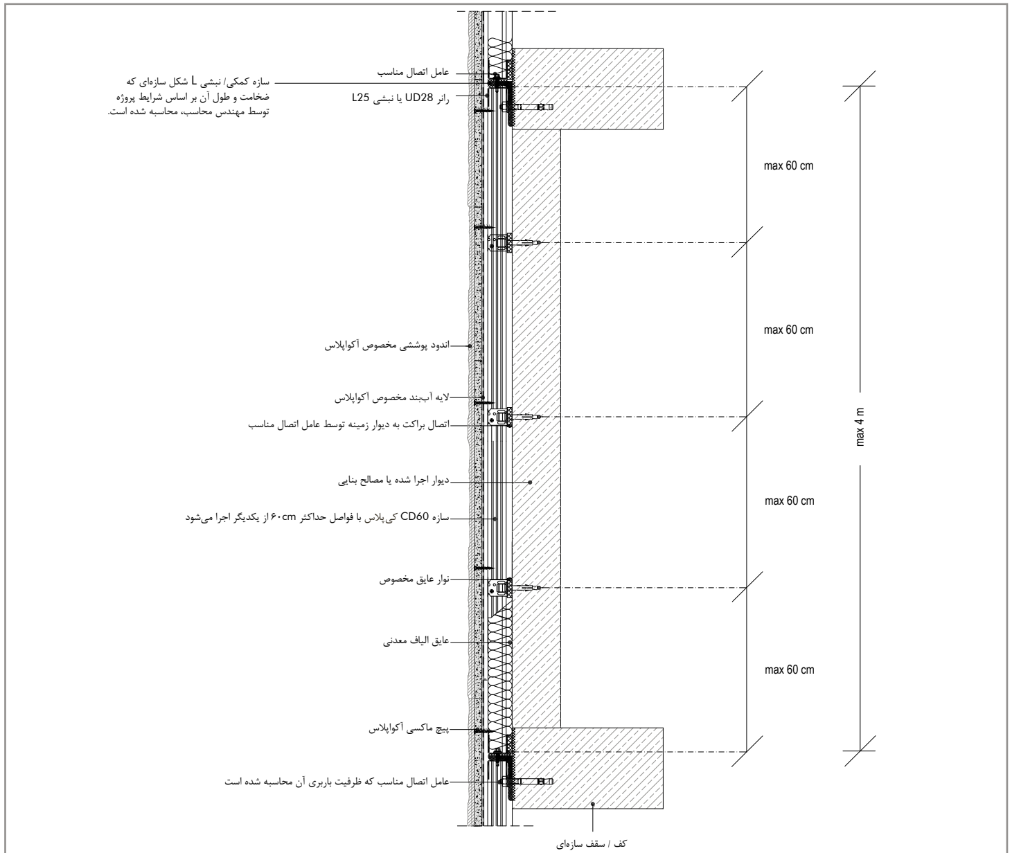
مقطع عمودی دیوار خارجی پوششی آکوپالاس با استفاده از سازه CD60
