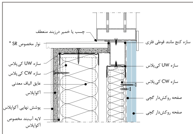
W388E-FE - VU1 گزینه ۱: اتصال دیوار خارجی آکوپالاس به قاب پایین پنجره
