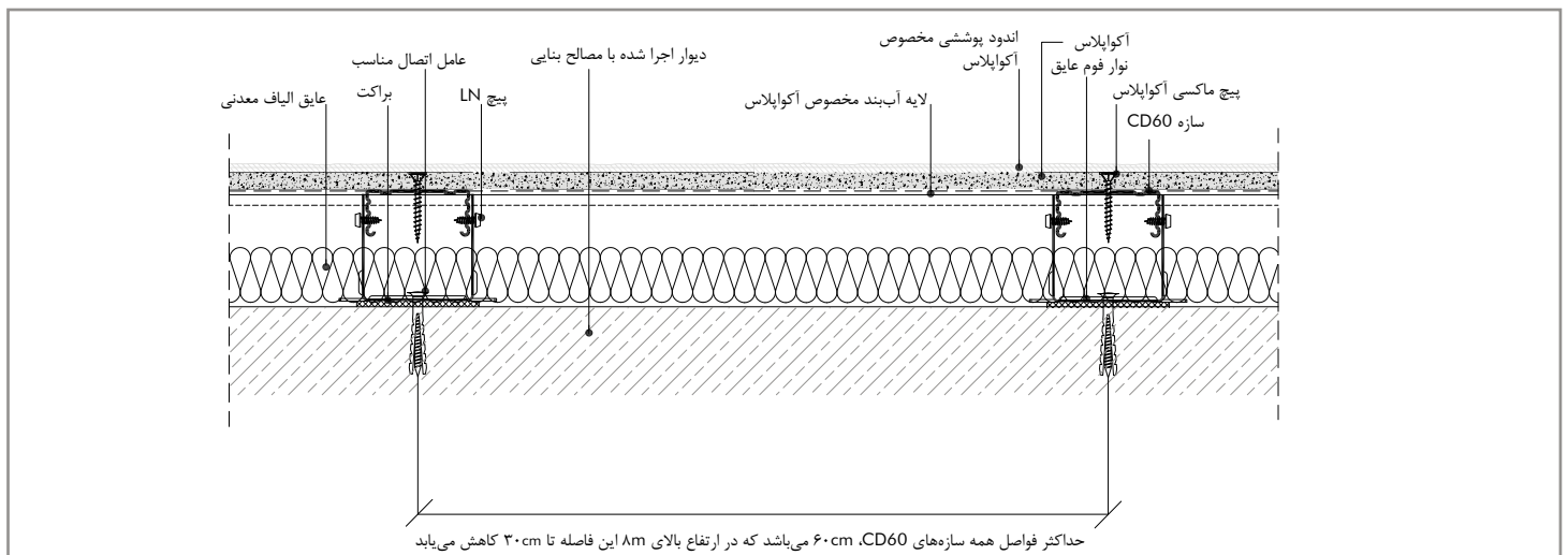
پلان دیوار خارجی پوششی آکوپالاس با استفاده از سازه CD60
