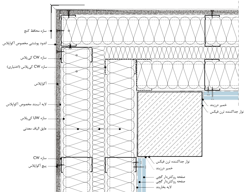
W388E-ES1 اتصال کنج خارجی سطح مقطع افقی
