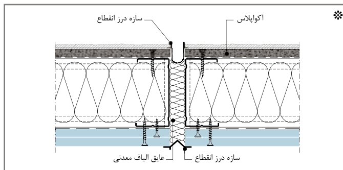
W384E-BF2 درز انقطاع سازه‌ای در دیوار
