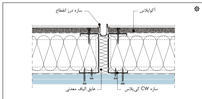
W384E-BF1 درز انقطاع در نما
