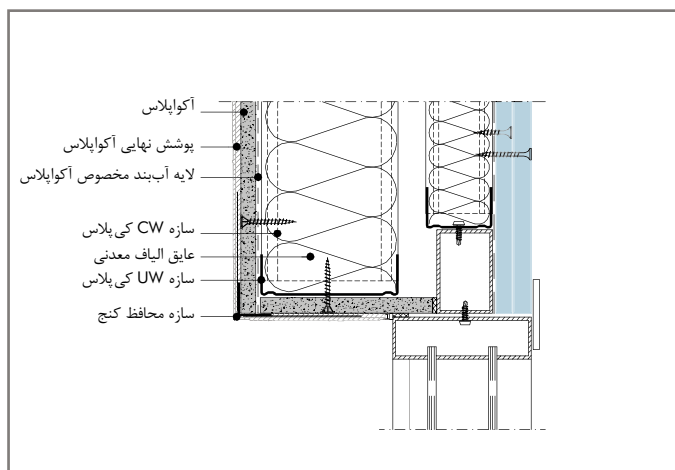
W388E-FE - VO1 گزینه ۱: اتصال دیوار خارجی آکوپالاس به قاب بالای پنجره
