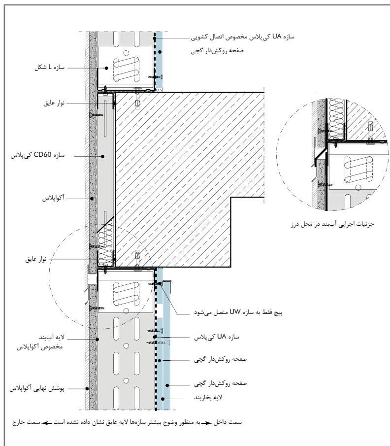
W384E-VMG2 گزینه ۲: اتصال کشویی لغزان به سقف سازه‌ای
