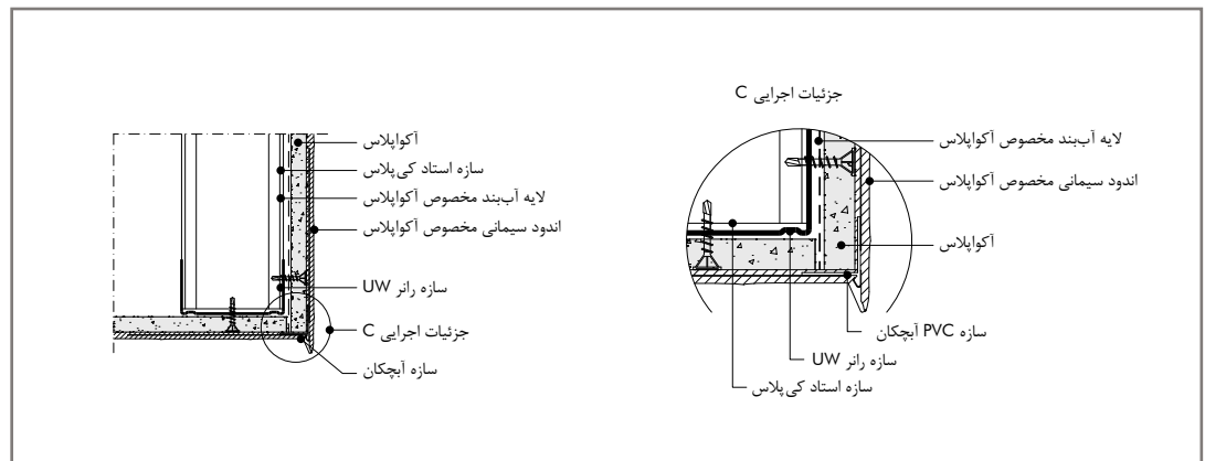
سازه مخصوص انتهای اندودکاری (آبچکان) از جنس PVC
