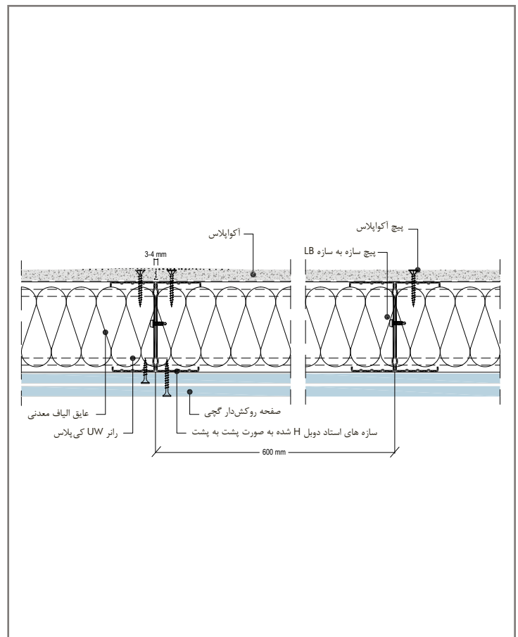
پلان دیوار خارجی آکوپالاس با استفاده از سازه استاد CW دوپل H
