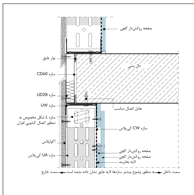
W384E-VMG1 گزینه ۱: اتصال کشویی لغزان به سقف سازه‌ای
