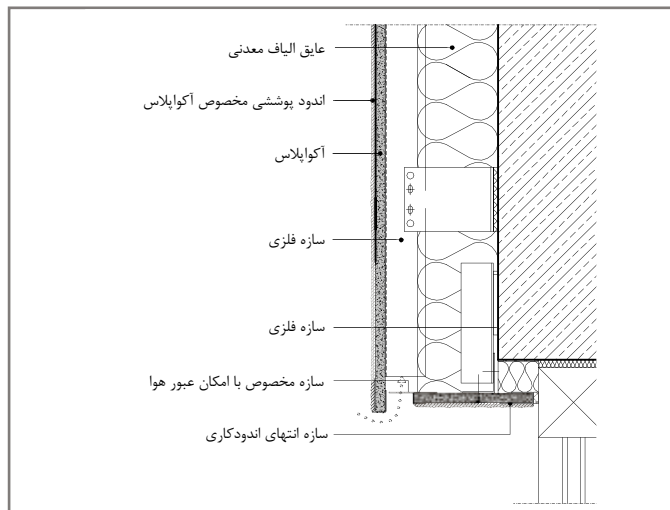
W684-FE - VO1 نحوه اتصال به قاب بالای پنجره
