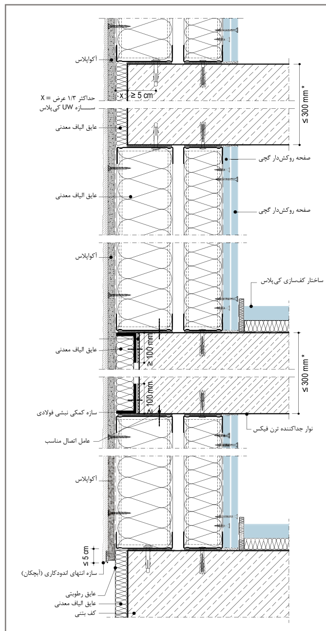
W388E-V1 مقطع عمودی
