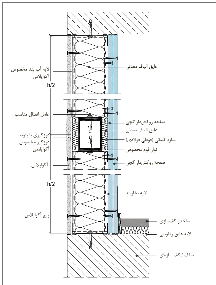
مقطع عمودی دیوار خارجی آکوپالاس با استفاده از قوطی کشی فلزی در وسط ساختار
