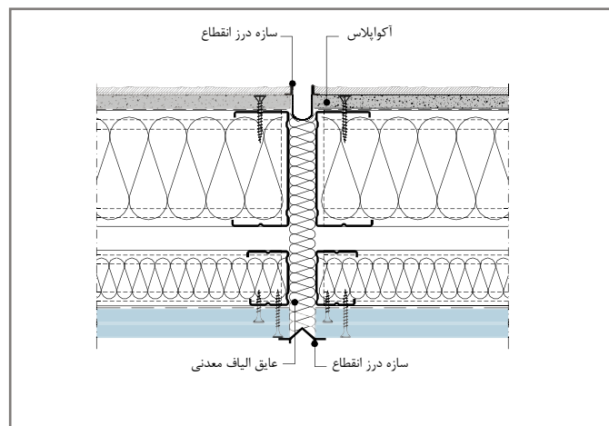
W388E-BFU1 درز انقطاع سازه‌ای
