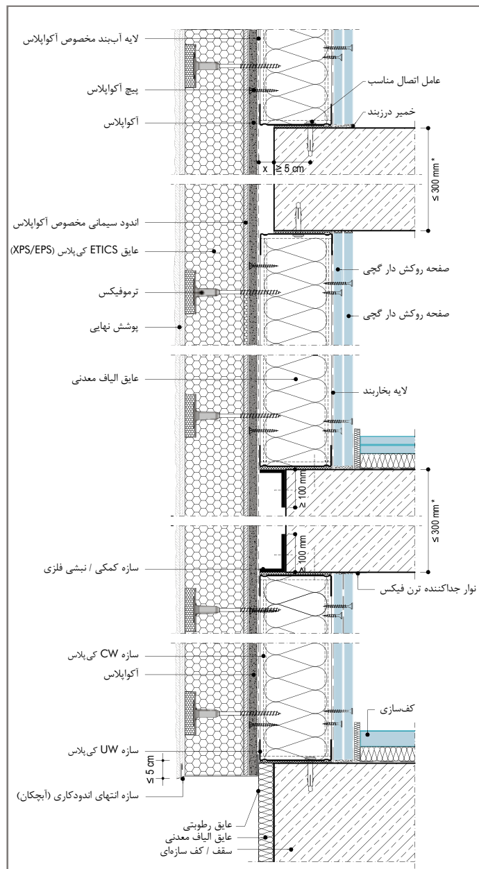
ETICS1 - V - W384E: سطح مقطع عمودی دیوار خارجی با ساختار ETICS
