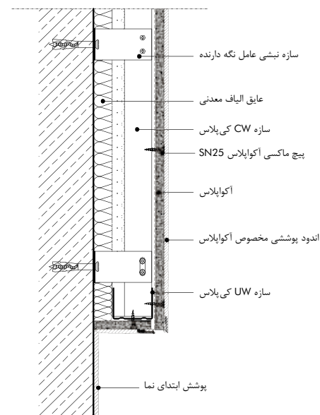
W684T-SO - V2 گزینه ۱: قسمت انتهایی کار دو نما (نقطه شروع)
