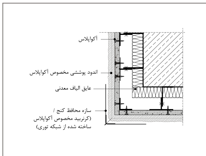
W684T-E1 نحوه اتصال کنج خارجی
