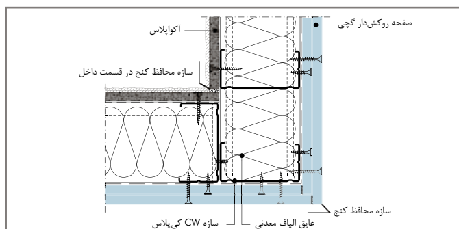
W384E-D1 اتصال کنج داخلی
