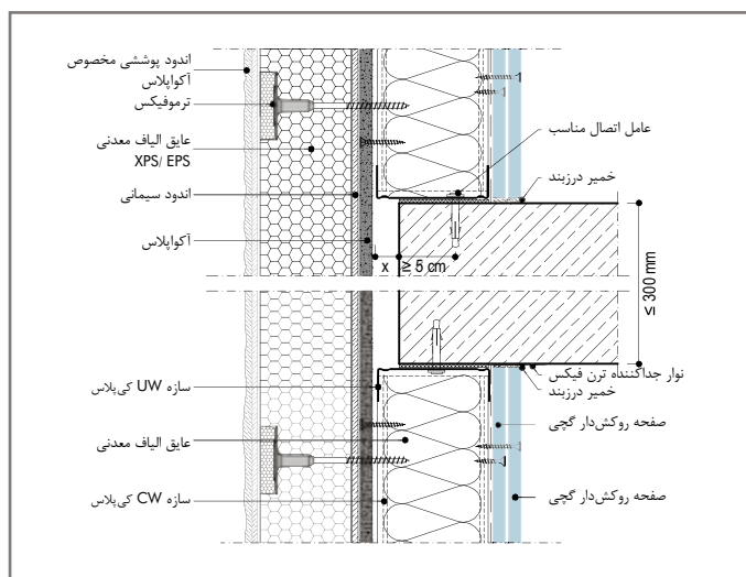
ETICS1 - VM - W384E: سطح مقطع دیوار خارجی با ساختار ETICS در تراز طبقه
