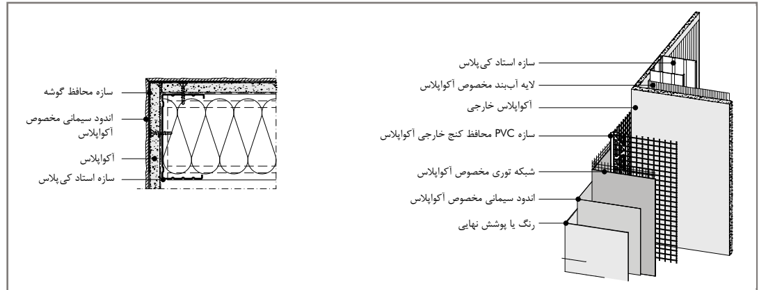
اتصال کنج خارجی با سازه PVC مخصوص
