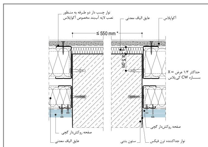
W388E-HS1 اتصال به ستون
