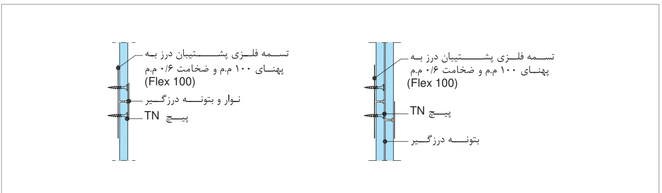
جزئیات درزگیری و اتصال لبه‌ها با تسمه فلزی پشتیبان
