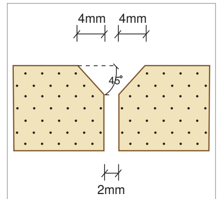
یک درز با دوبله پخ خورده
