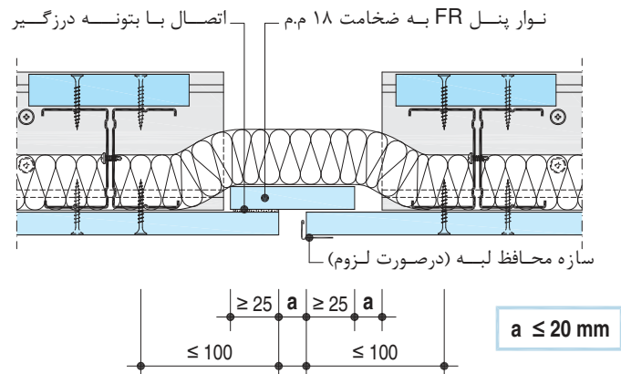
درز انقطاع با اتصال کشویی لغزان (سقف کاذب خود ایستا با کد حریق ۳۰ دقیقه از پایین و بالای سقف کاذب - تیپ A)
