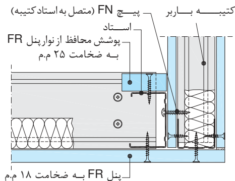
اتصال سقف کاذب خود ایستا به کتیبه باربر
