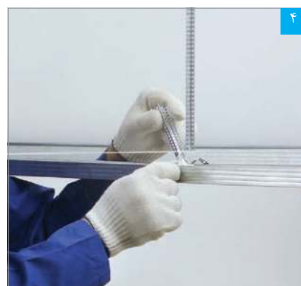
استقرار چنگک
