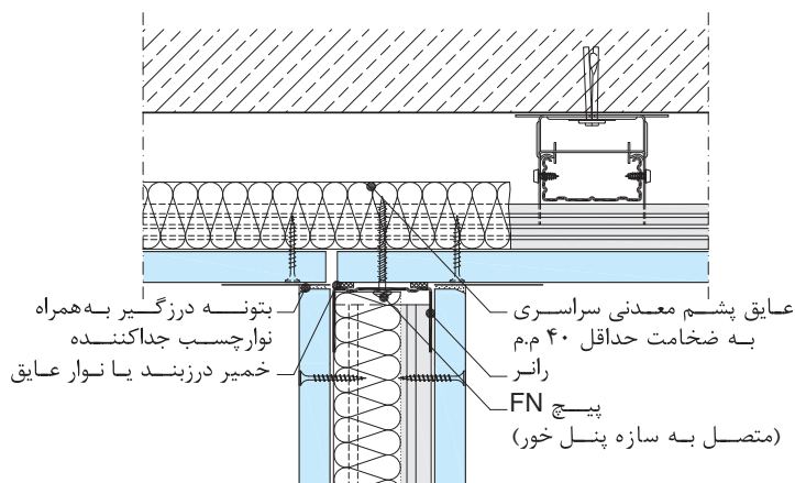
اجزای بادبندی سقف
