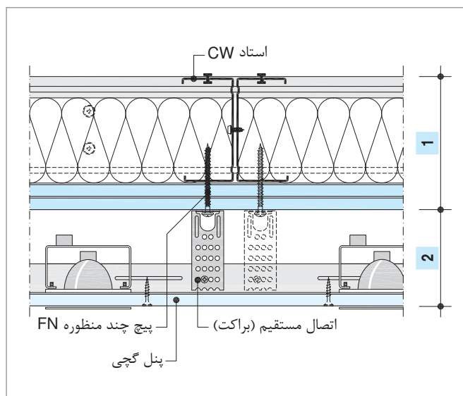
جزئیات اجرایی
