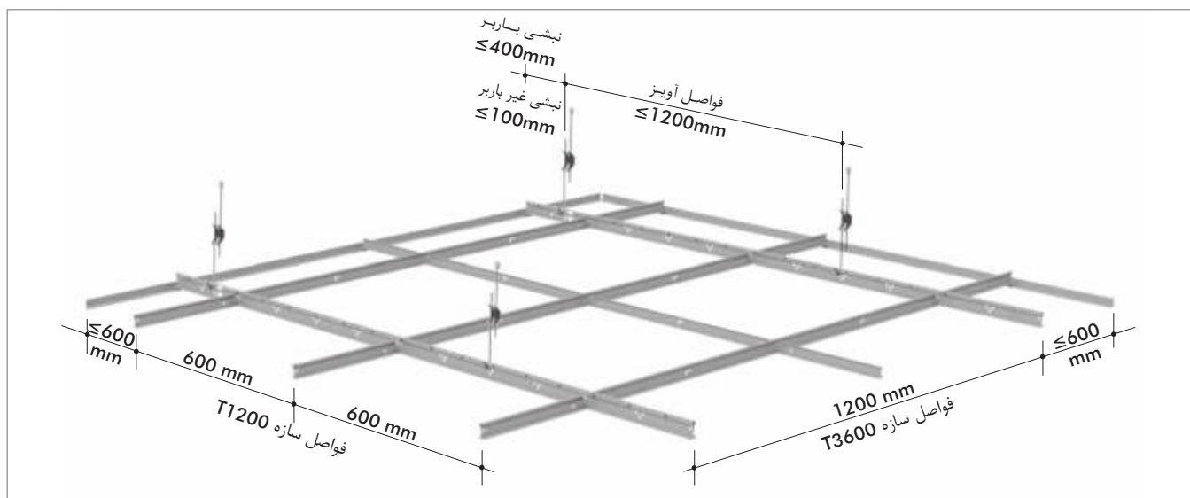
فواصل سازه‌ها و آویزها
