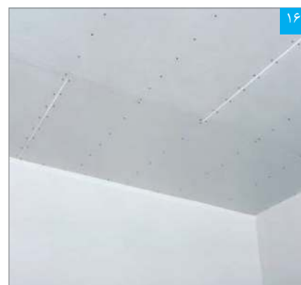
پتل‌گذاری تکمیل شده (به صورت حصیرچین)
