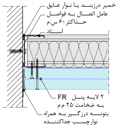
اتصال دیوار پوششی W628b به دیوار بنیایی جانبی (۲×۲۵) W628b-11
